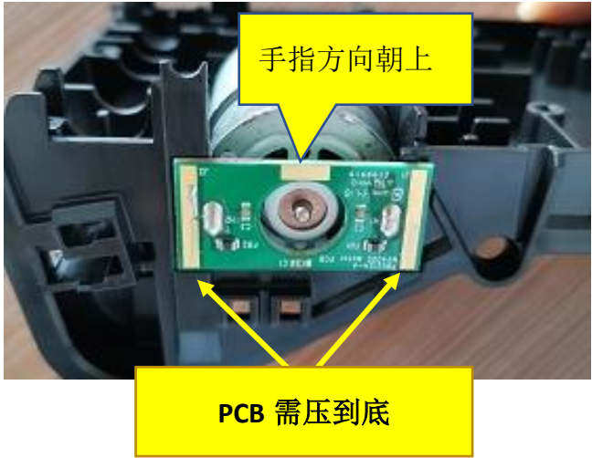
图二, 装入马达组件 PA3295 时, 板子上中间手指方向朝上装入 PA3299-3 并装到位 (如图示)
