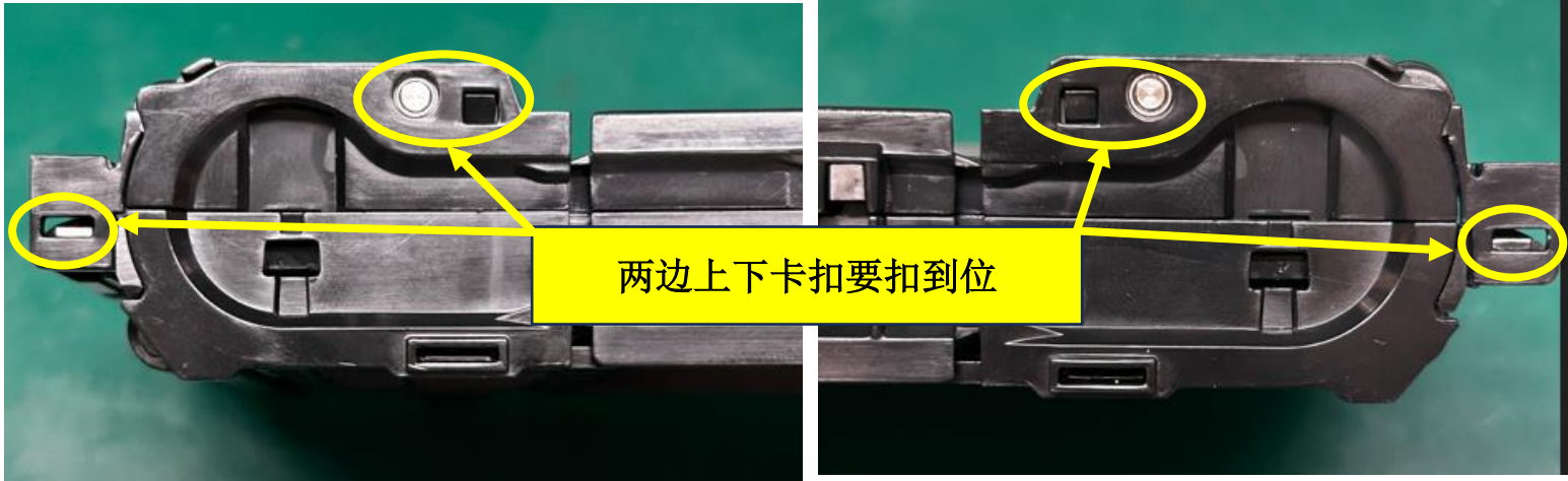
图二、将图一装好的组件装入 PA03040-1,注意两边上下卡扣要卡到位。
