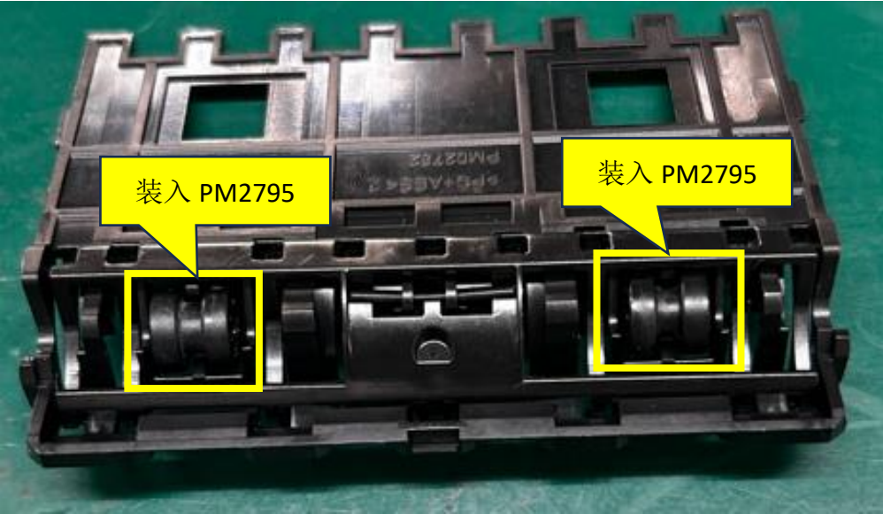
图一，将 2 个 PM2795 装入 PA3037-1 组件两边的槽位。
