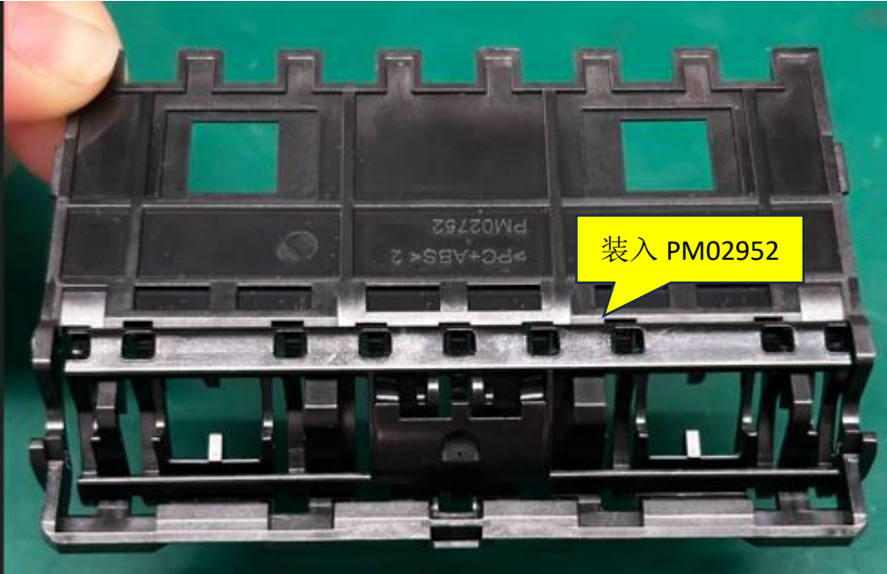
图一，将 PM2952 装入 PM2752 槽位里面。
