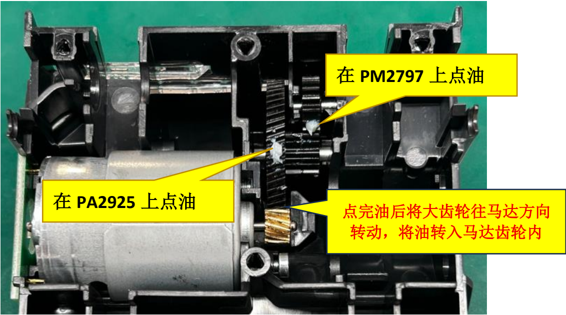
图一、用点油机在 PA2925 和 PM2797 齿轮位置加上大约 0.007g 的润滑油。
