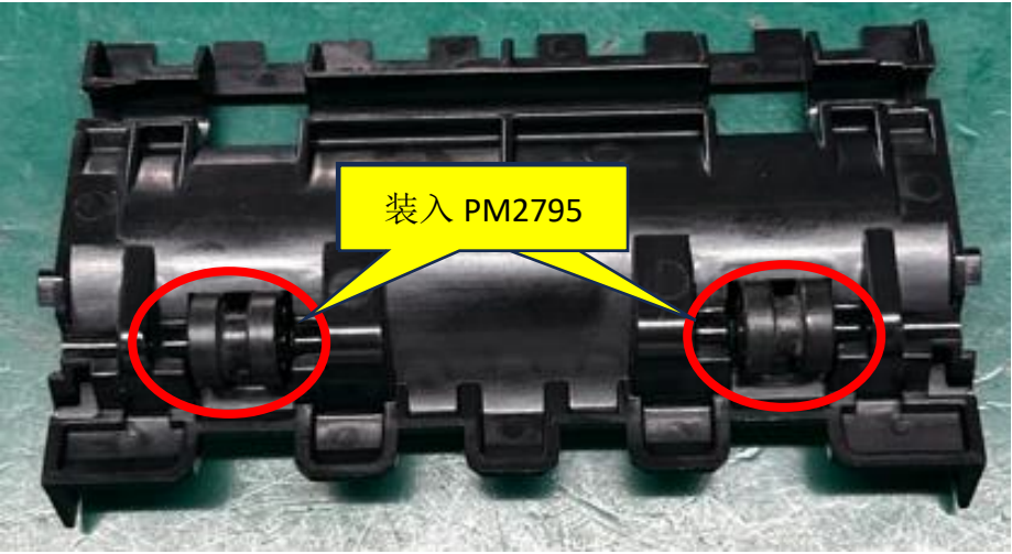
图一，将 2 个 PM2795 装入 PM02751 两边的槽位。
