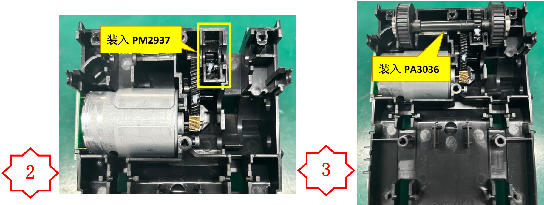
图二，将 PM2937 骨位对准胶件槽位朝下装在齿轮上方，装完后要与塑胶面平齐。
