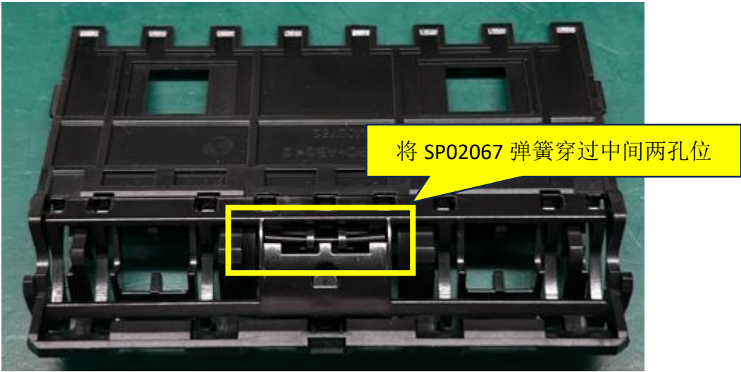
图二，将 SP02067 弹簧穿过中间两孔位，并将弹簧固定在槽位里面。
