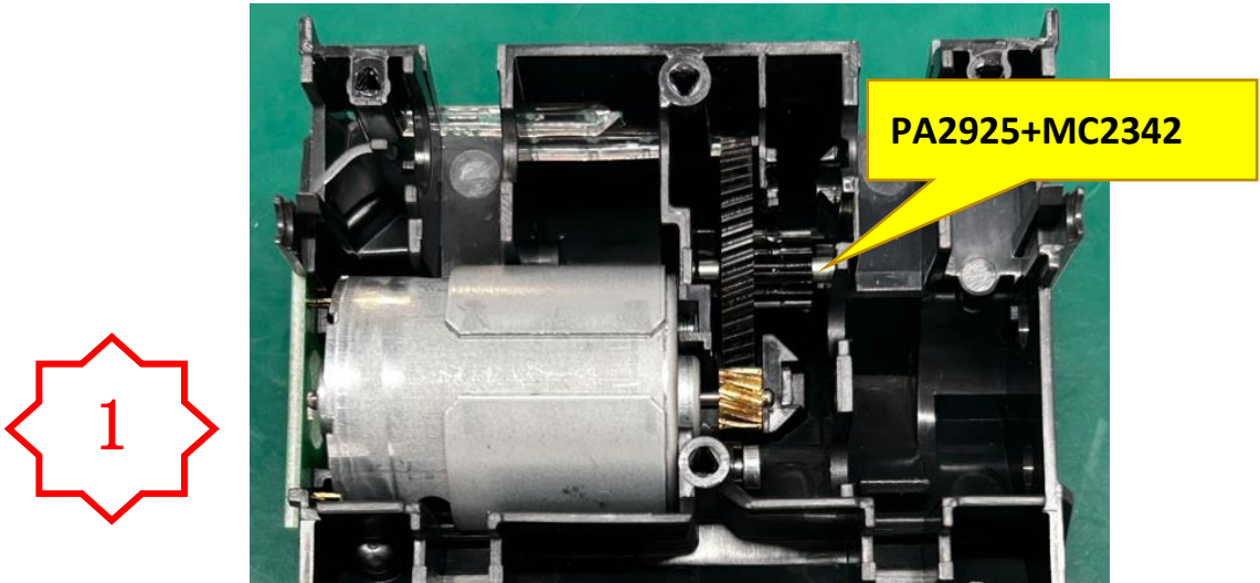
图一，装入 MC2342+PA2925 到对应的位置，注意装配到位。
