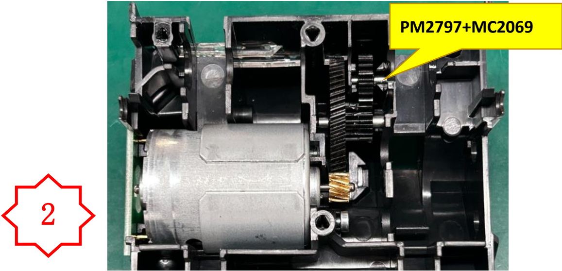
图一，装入 MC2069+PM2797 到对应的位置，注意装配到位。
