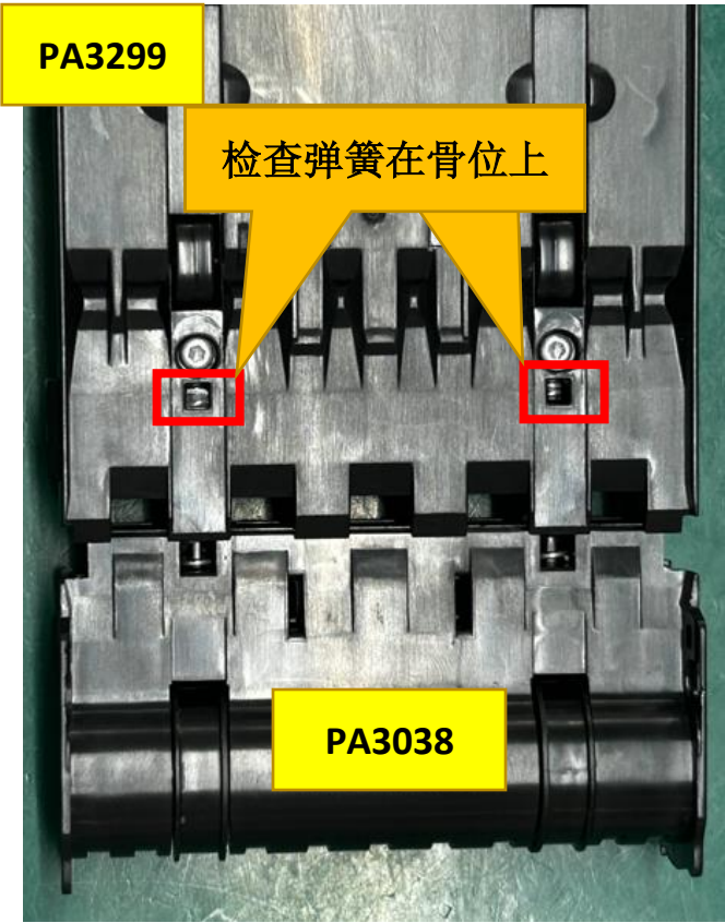
图一，将 2 个 SP2011 分别装在 PA3038 左右槽位，再装入 PA3299 组件，注意方向：PA3299 螺丝朝上,弹簧对准 PM2747 两边骨位装入，装到位后检查弹簧须在骨位上。
