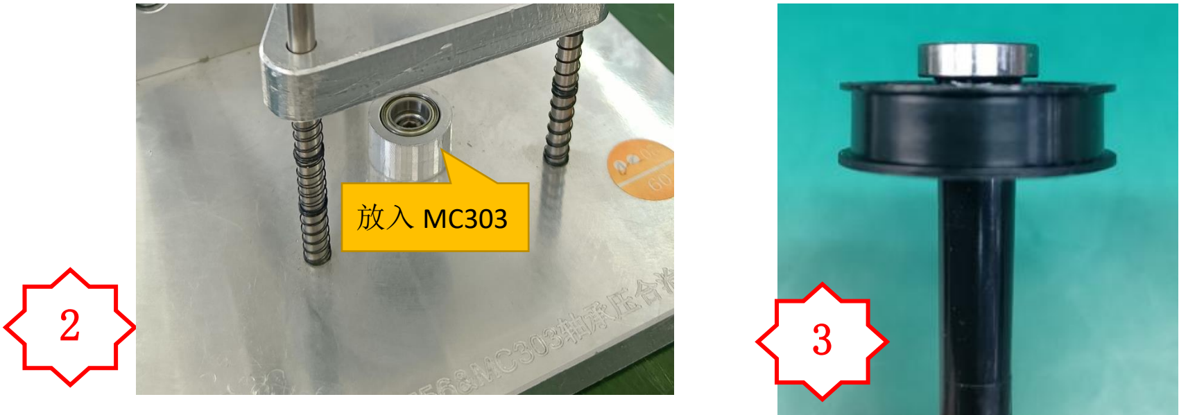
图二，把 MC303 放在治具的最下孔内，PM2756 短柱朝下放入治具上进行压合（如图二所示）
