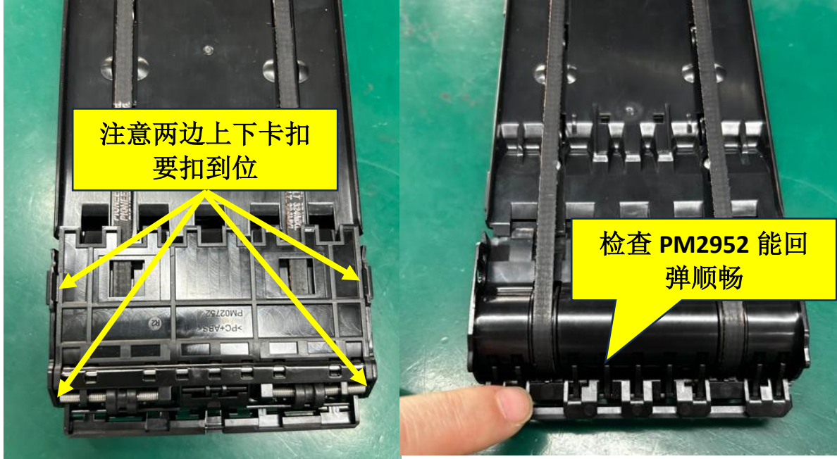
图二、将图一组件装入 PA3298,注意两边要扣合到位，检查 PM2952 能回弹顺畅。
