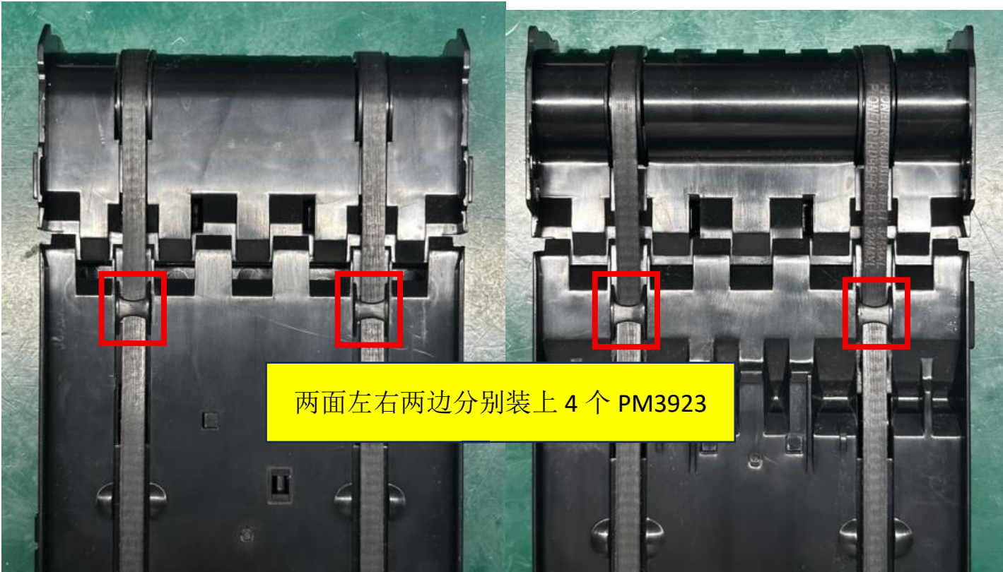
图一、在 PA3040 组件两面两边装皮带位置分别装上 4 个 PM3923。
