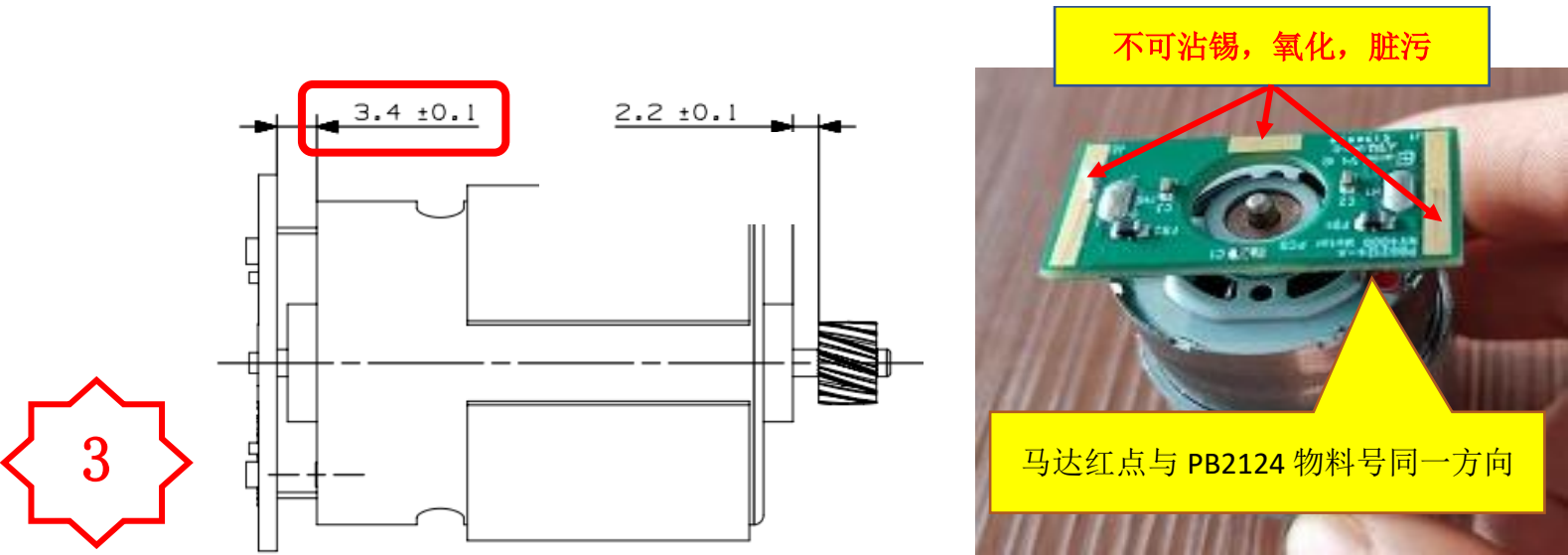
图三，确认 PCB 板与马达的方向正确后进行焊锡，焊好板子与马达间隙尺寸 3.4 \pm 0.1\text{mm} ，板子上金色连接器不可沾锡（如图示）
