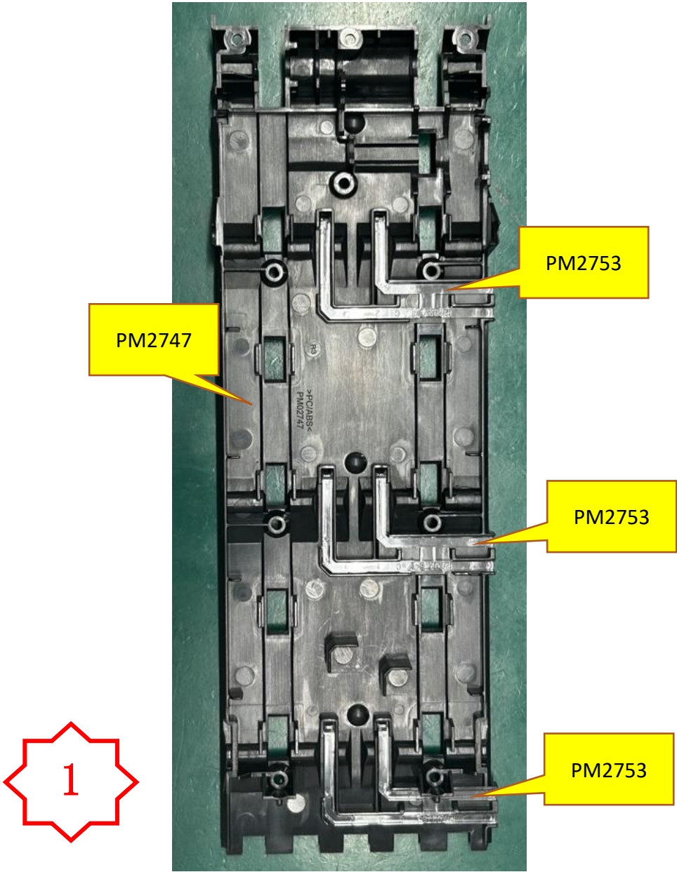
图一，将 3 个 PM2753 装在 PM2747 上，再放入压合治具上进行压合到位。
