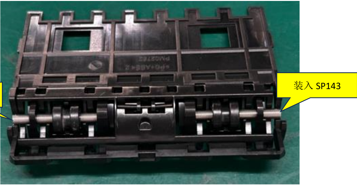
图二，将 2 个 SP143 弹簧从两边孔位装入，注意装配到位，弹簧不高出胶件两边的平面。
