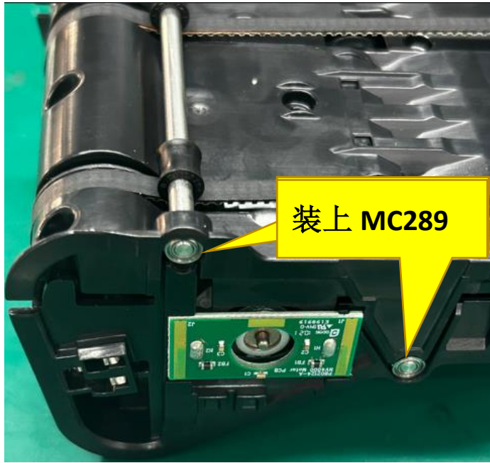
图二，在五金轴上分别装上 2 个 MC289，MC289 须在卡扣的里面。
