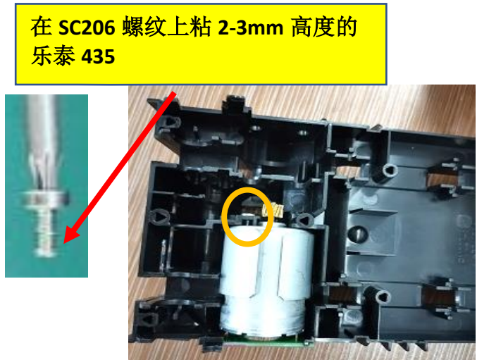
图四, 在 SC206 螺纹上粘 2-3mm 高度的乐泰 435 打在马达与 PA3299-3 短孔内 (如图示)
