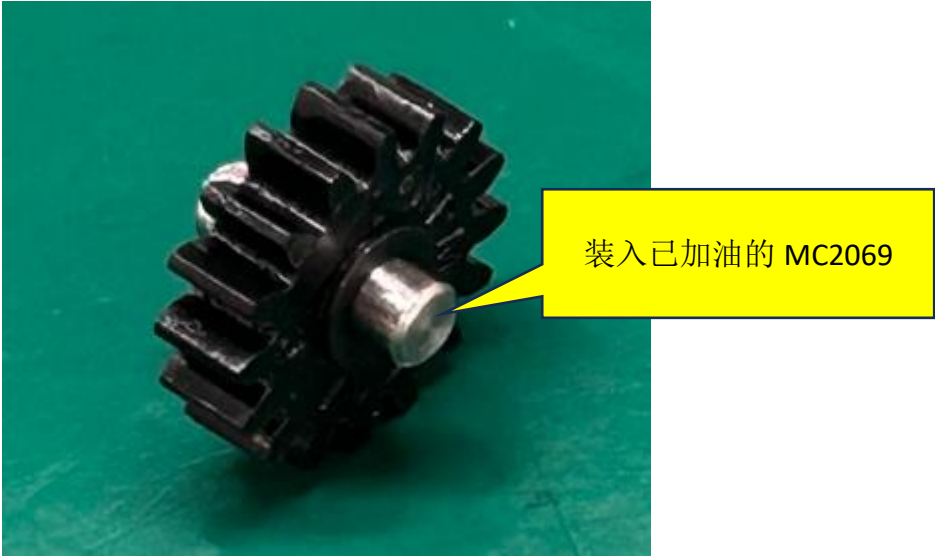
图一，在 PM2797 孔内装入点了油的 MC2069 五金轴。
