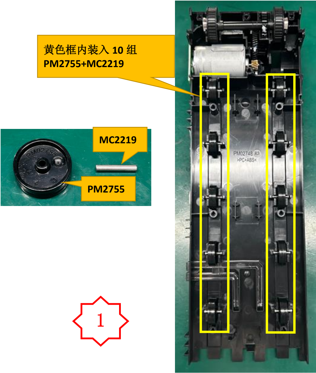
图一，将 MC2219 装入 PM2755 的孔内，再将其装入 PA3299-6 的槽内，共 10 组。
