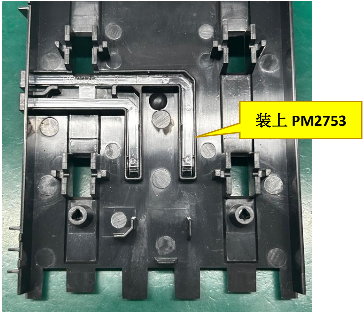
图二，将 PM2753 装在 PA3299-2 的 PM2748 上,再将装好组件放在治具上压合，将导光柱按压在塑胶件上面贴紧。
