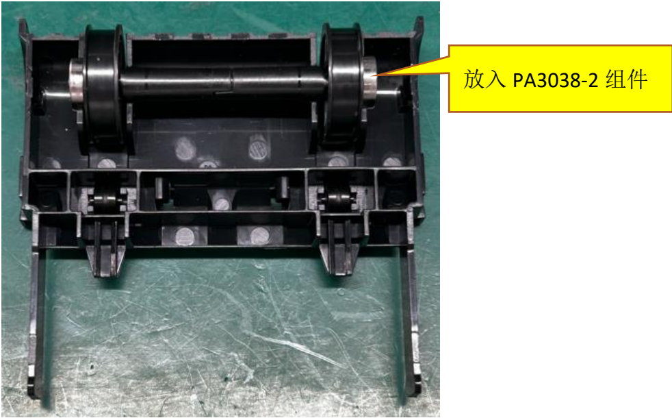
图一，在 PA03038-3 组件槽位放入 PA3038-2 组件。
