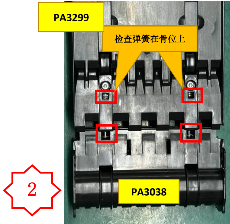
图二，PA3299 组件螺丝朝上将 PA3038 装入，弹簧对准 PA03038 两边骨位装入，检查弹簧须在骨位上。
