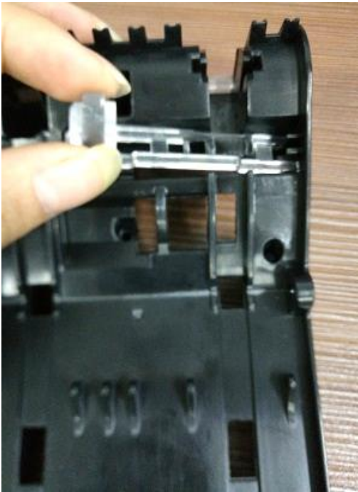
图二，将 PM2793 柱子朝上装在 PA3299-1 的 PM2748 上,将导光柱左边骨位推入 PM2748 扣位里面。（如图示）
