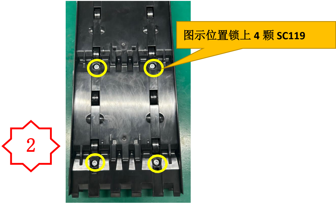
图二，在图示位置分别打入 4 颗 SC119 的螺丝。
