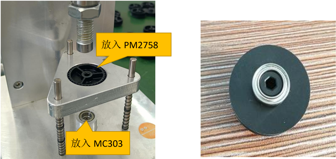
图二，将 MC303 与 PM2758 分别放进治具，压入 PM2758 的柱子上，压完后与柱面平齐（如图示）
